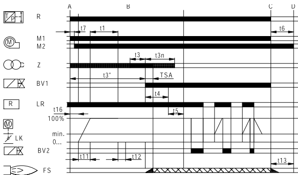
Двухступенчатая горелка
